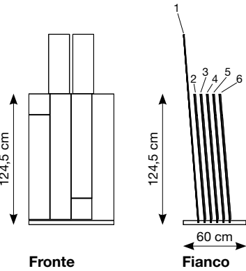
EXPO STEP 80 OAKS 81x60xh124,5 cm Base culla (vuota) PBEA
