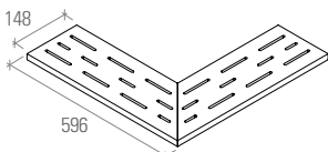
Angolo griglia 15x60
