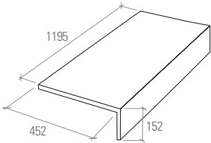
Terminale "L" 120x45x15
