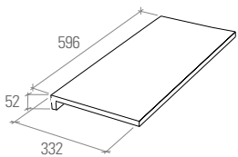
Scalino Incollato 33x60x5
