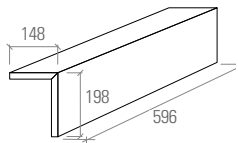
Cordolo "L" 60x20x15
