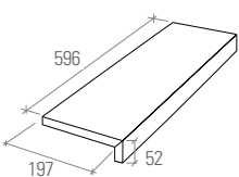
Terminale "L" 60x20x5
