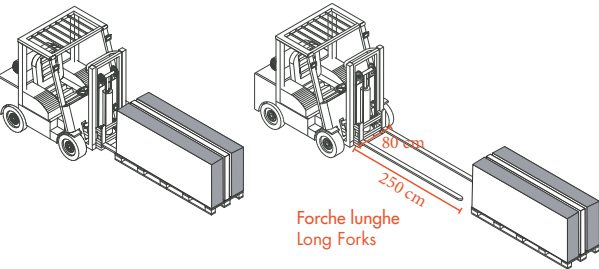
Carico su Container Container loading
